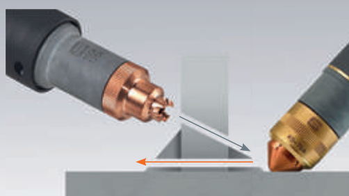
COUPE STANDARD
