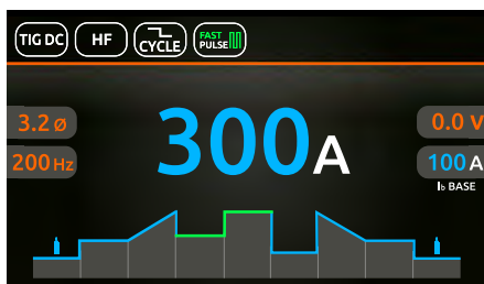
MODALITA' SALDATAURA
