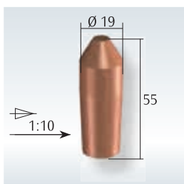
Electrodo standard
