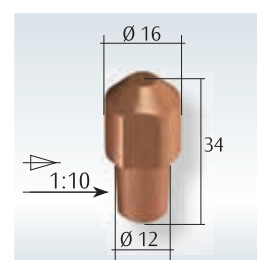
Elettrodo per braccio inferiore ad ingombro ridotto
